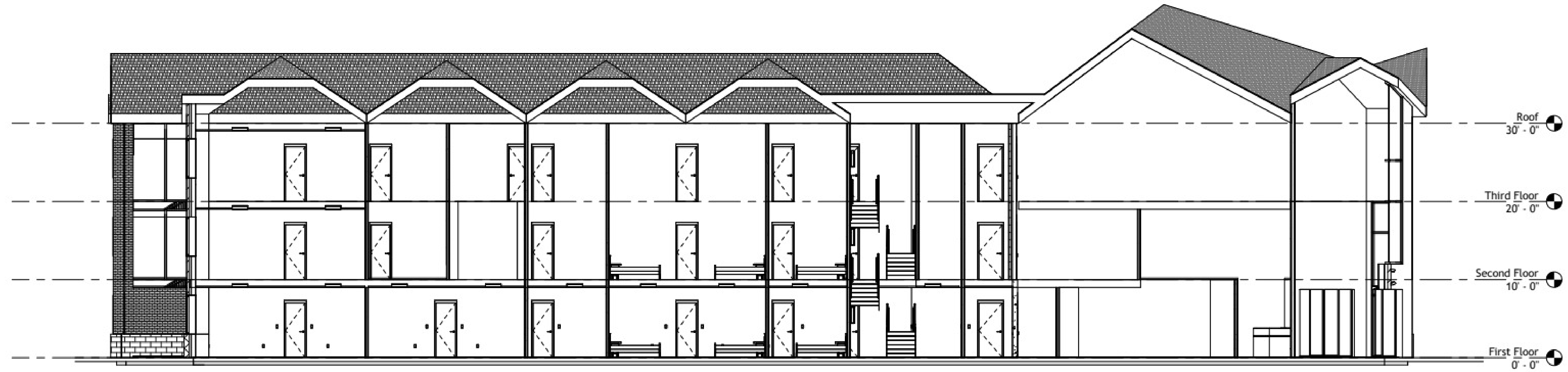
① East Longitudinal Section 1/8" = 1'-0"
